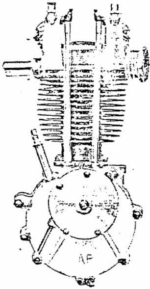
250 c.c. Culbuteurs "STANDARD" 1 ou 2 échappements
