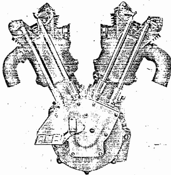
1.100 c/c. Culbuteurs "RACING"
