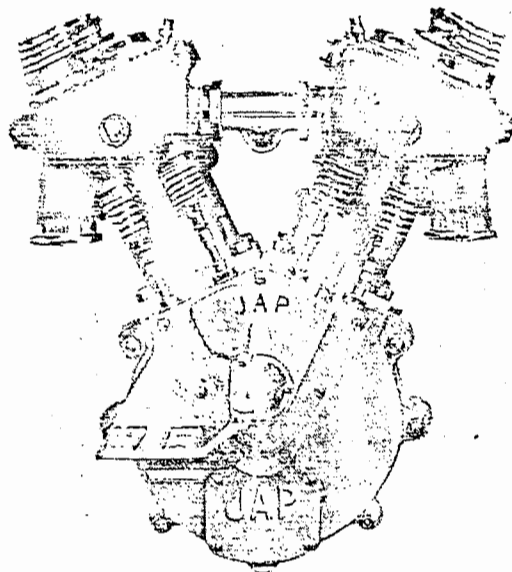
1.000 c.c. Soupapes Latérales "STANDARD A EAU"
