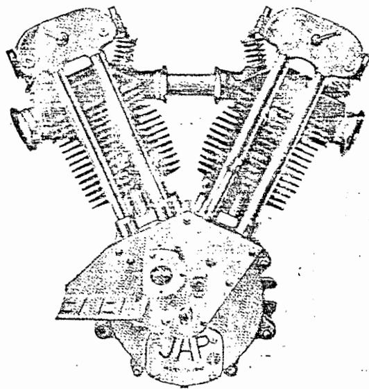
680 ou 1.000 c.c. Culbuteurs "STANDARD"
