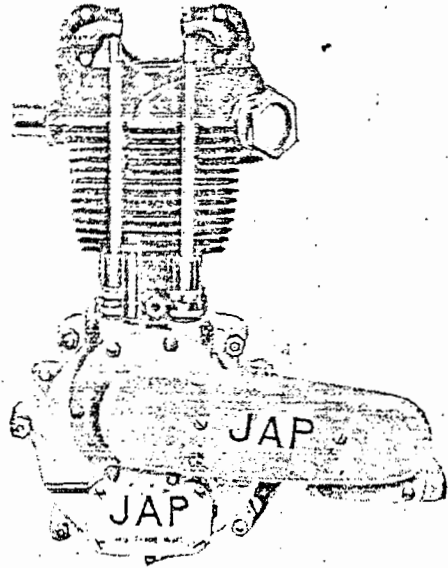
250 c.c. Culbuteurs "RACING"
