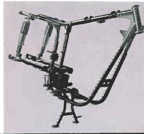
Cadre en double berceau d'une rigidité absolue. Fourche avant télescopique, suspension arrière oscillante avec amortisseurs.
