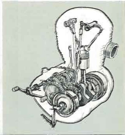
Transmission primaire par engrenages hélicoïdaux parfaitement silencieux. Boîte à 4 vitesses avec point mort verrouillé.
