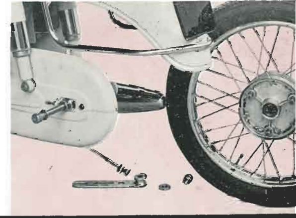
Roue arrière facilement démontable grâce à son moyeu broche. Freins à tambour central, rayonnage renforcé, amortisseur de transmission.
