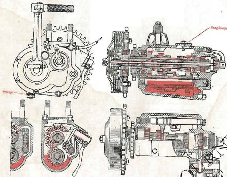
Fig. - Boîte 3 vitesses
