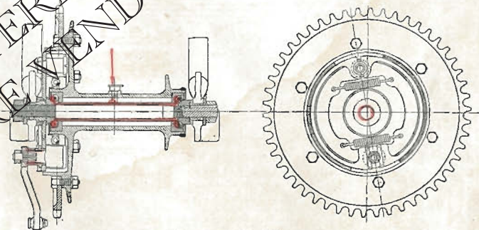
Moyeu et frein AR
