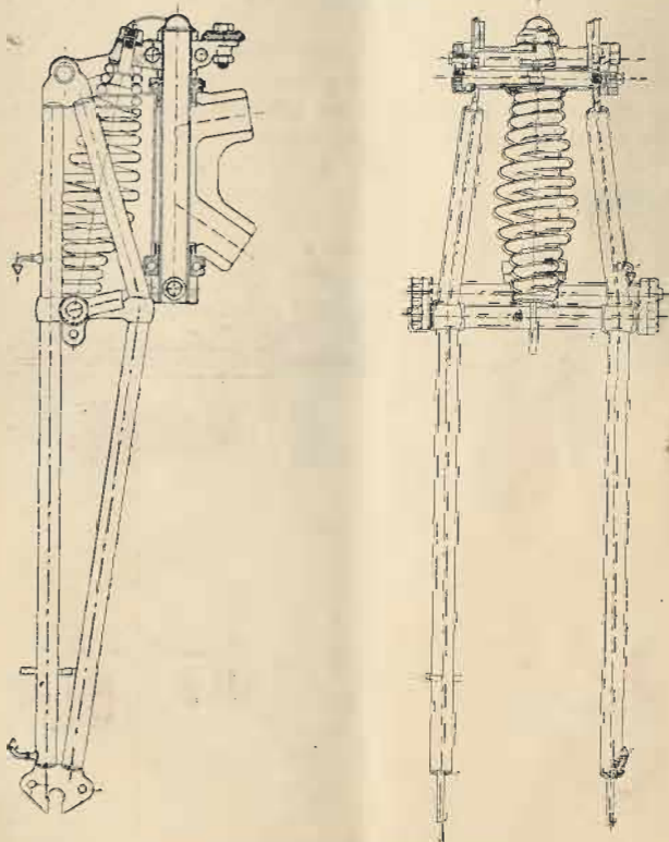
Fourche de 120 m/m ressort central.
