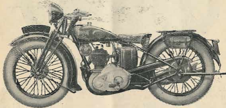
500 cc. 4 temps MONOBLOC Type RL. graissage par pompe mécanique à circulation continue et carter sec.
