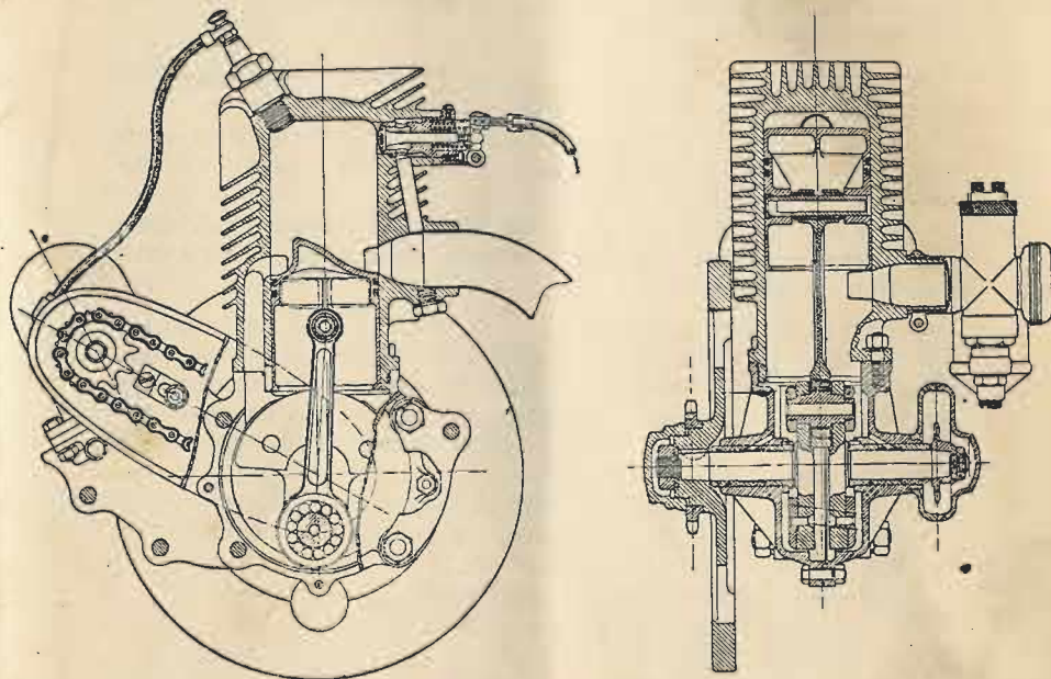
Moteur 250 cc. 2 temps
