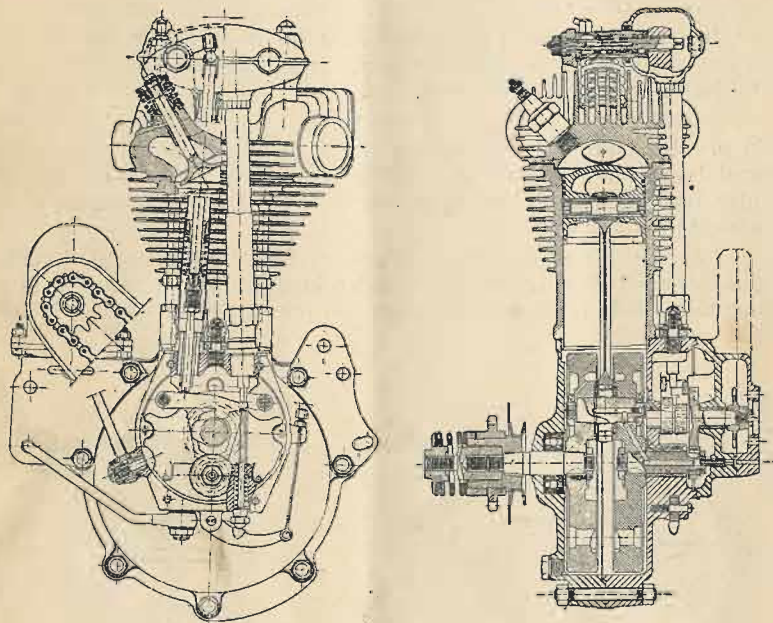
Moteur 350 cc. culbuteurs.
