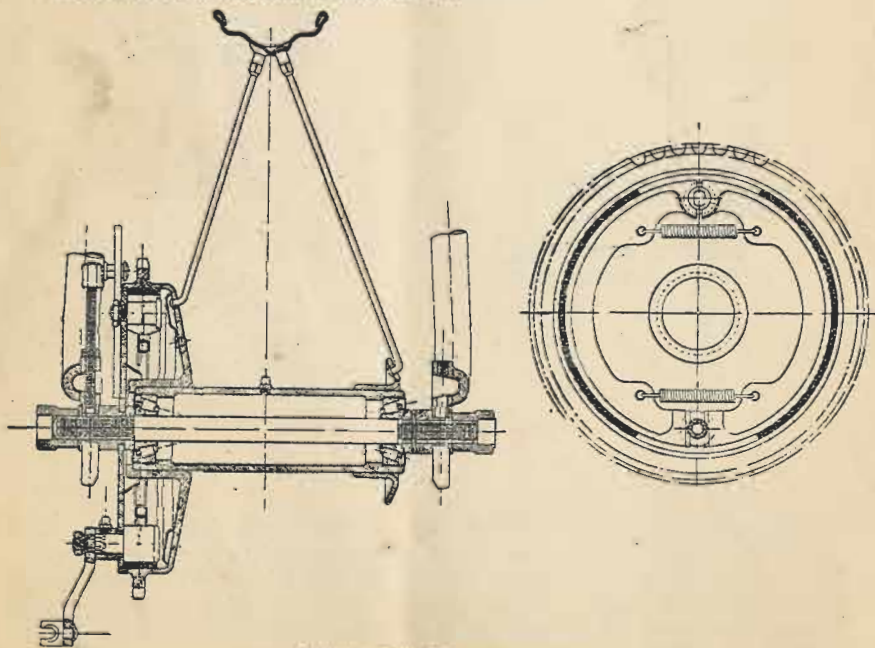
Moyeu à roulements « Timken ».
