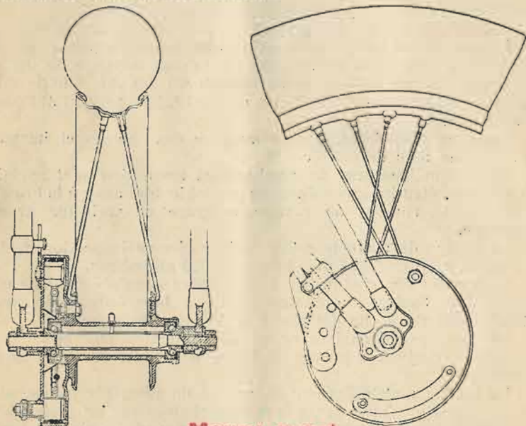
Moyeu avant
