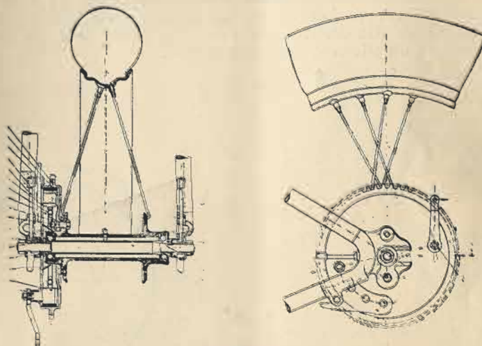
Moyeu arrière
