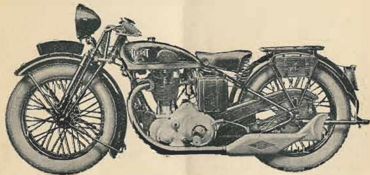
4 temps supersport, type HR, pompe Pilgrim à circulation continue et carter sec.
