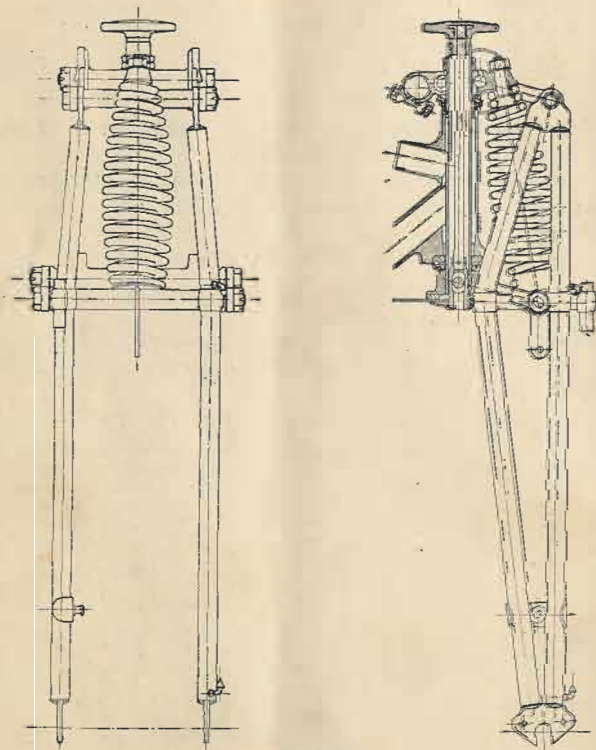
Fourche élastique. Fourche élastique de motocyclette 350 cc., type HLG.
