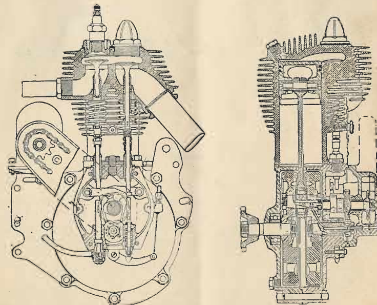
Moteur 350 cc. Standard.
