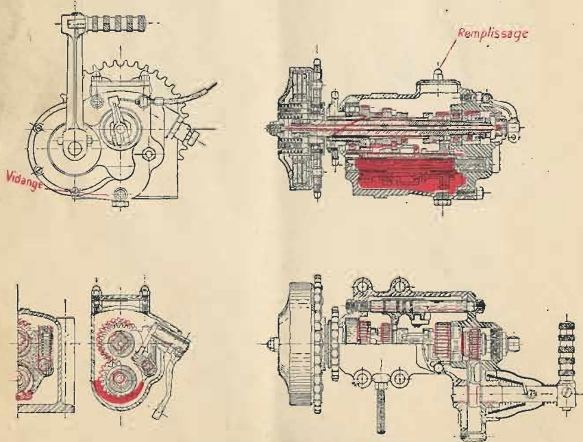
Fig. 4. — Boîte 3 vitesses TERROT.
