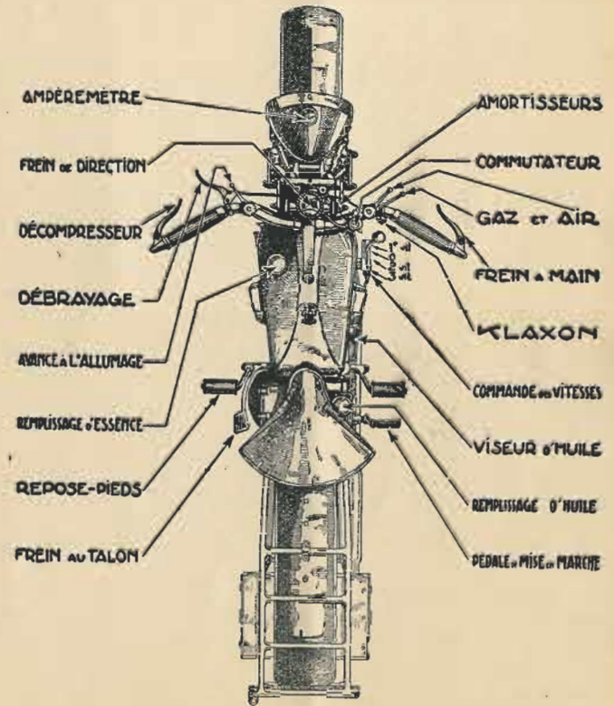
Vue en plan de la Motocyclette 350 cc. Standard montrant la disposition des commandes
