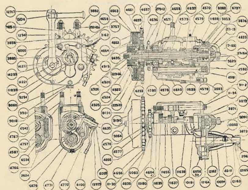
Boîte 3 vitesses TERROT.
