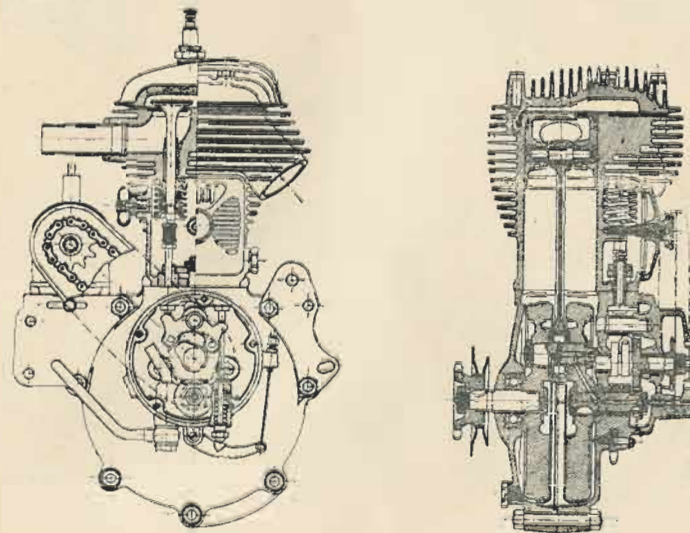
Moteur 350 cm 3 à soupapes latérales.
