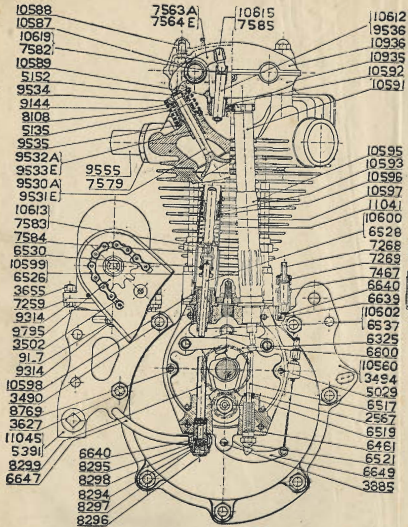
Moteur 250 CC., type MOSSE
