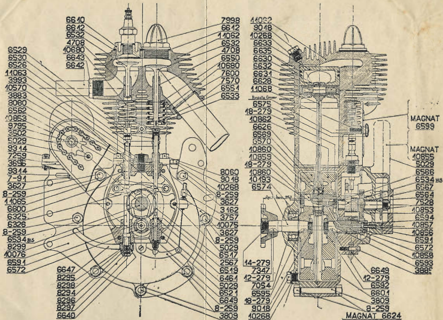
Moteur 350 CC., type B0. BST graissage central.
