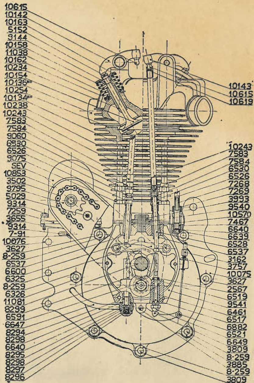
TEPROT Moteur 350 CC., type HSSO, graissage central.
