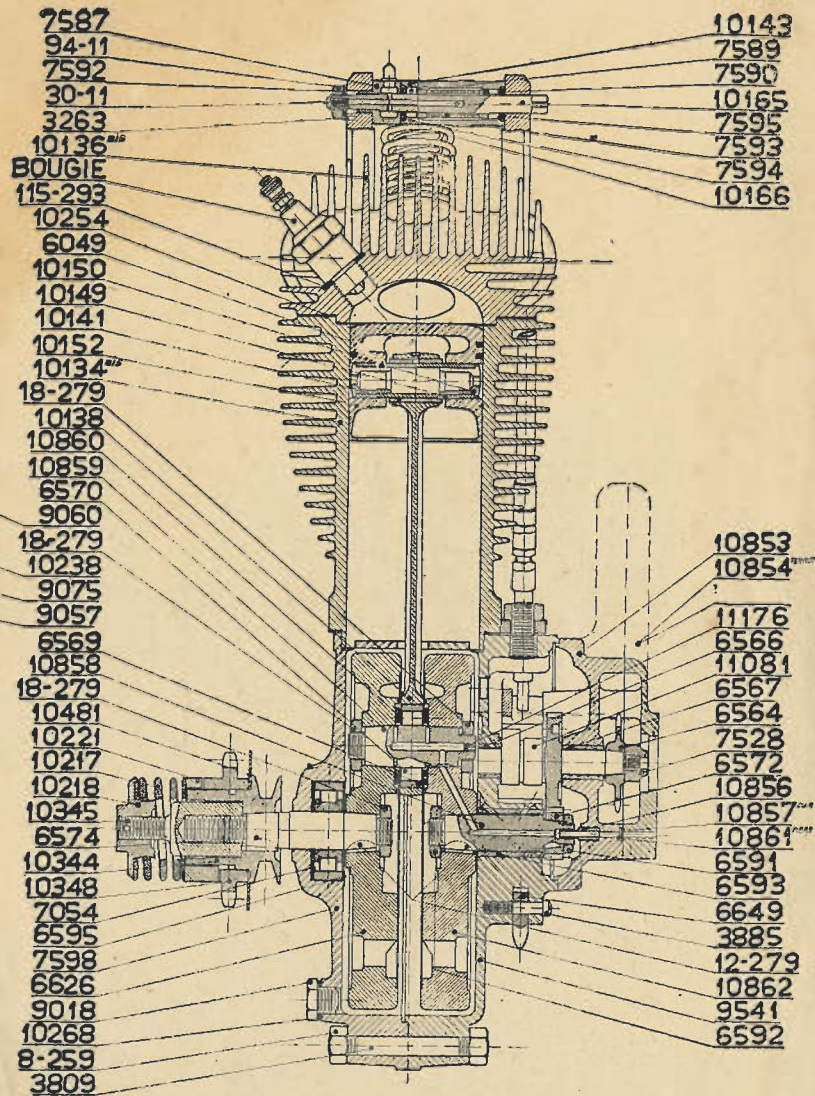
TEPROT Moteur 350 CC., type HSSO, graissage central.
