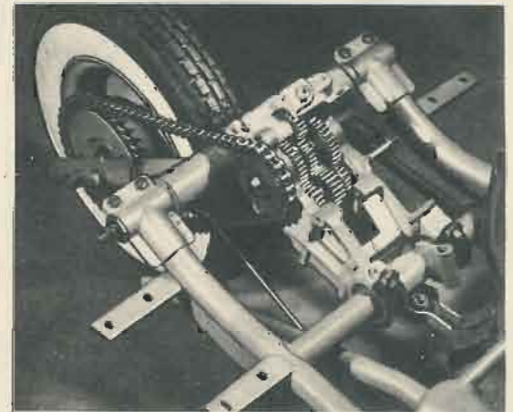
Détail de la boîte présélective
